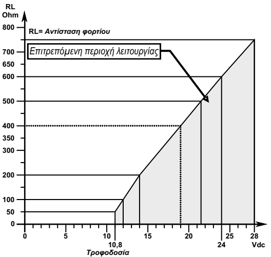
Σχήμα 4 Διάγραμμα τροφοδοσίας/αντίστασης φορτίου 4 ±20mA
