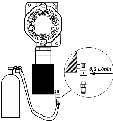
Σχήμα 3 Ελεγκτής ρύθμισης
